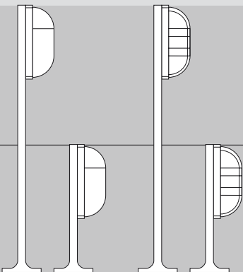
Alu-Lux oval
